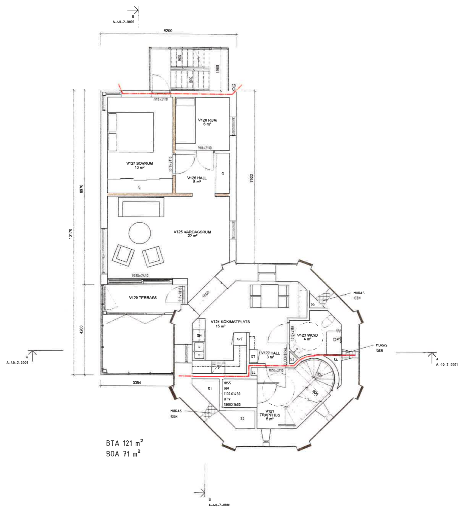
PLAN 12 ÖVERSIKT 1 : 50
